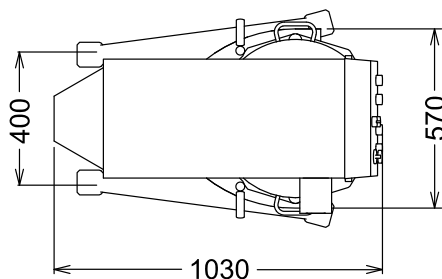
Boven aanzicht
